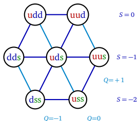
Quark Modeli — 1964
