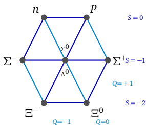
Baryon Okteti — 1961
